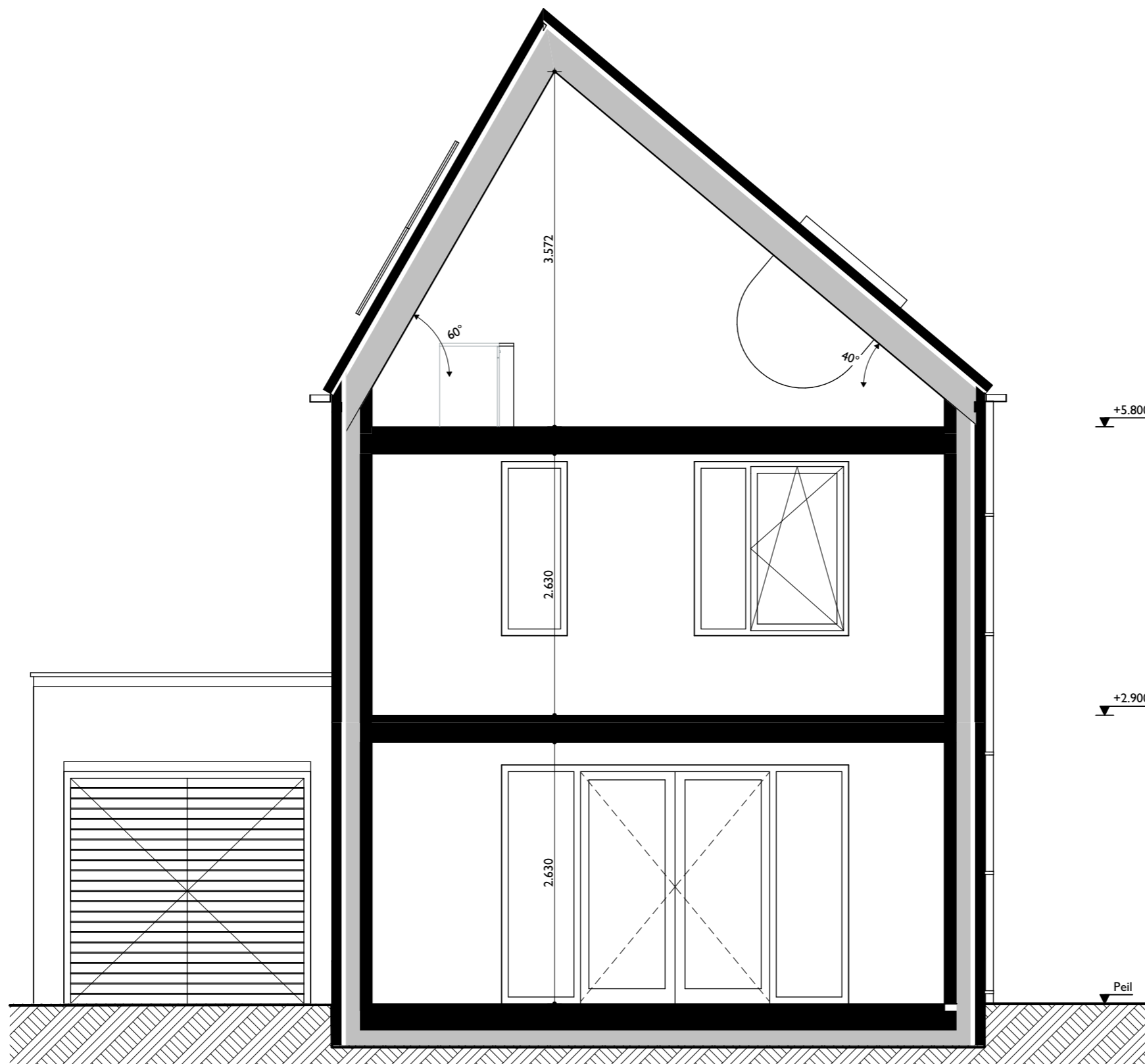
Doorsnede A-A
