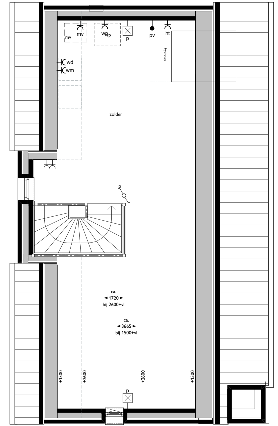
02 tweede verdieping
