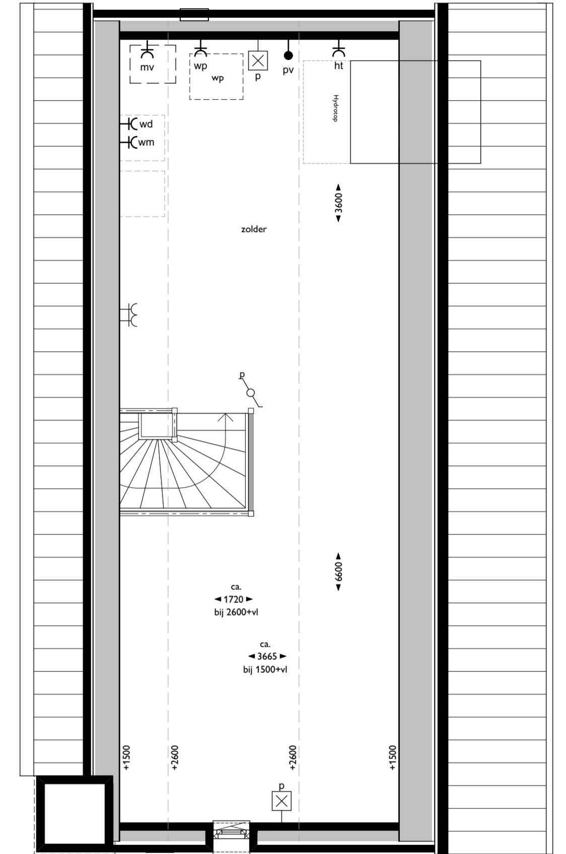
02 tweede verdieping
