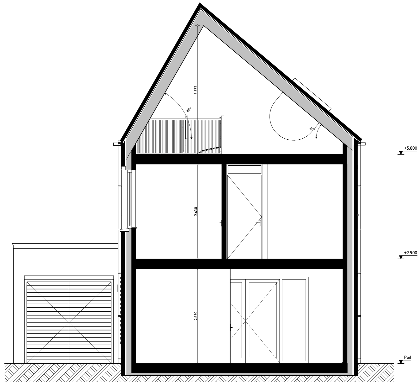
Doorsnede A-A
