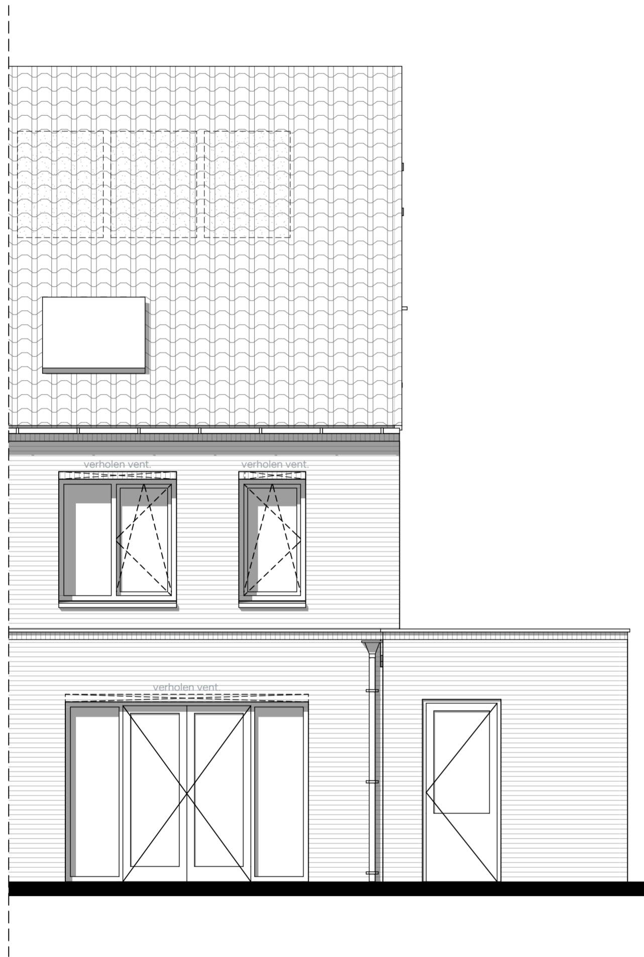
Achtergevel
