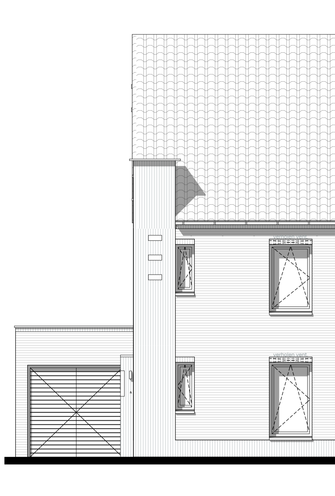
Voorgevel
