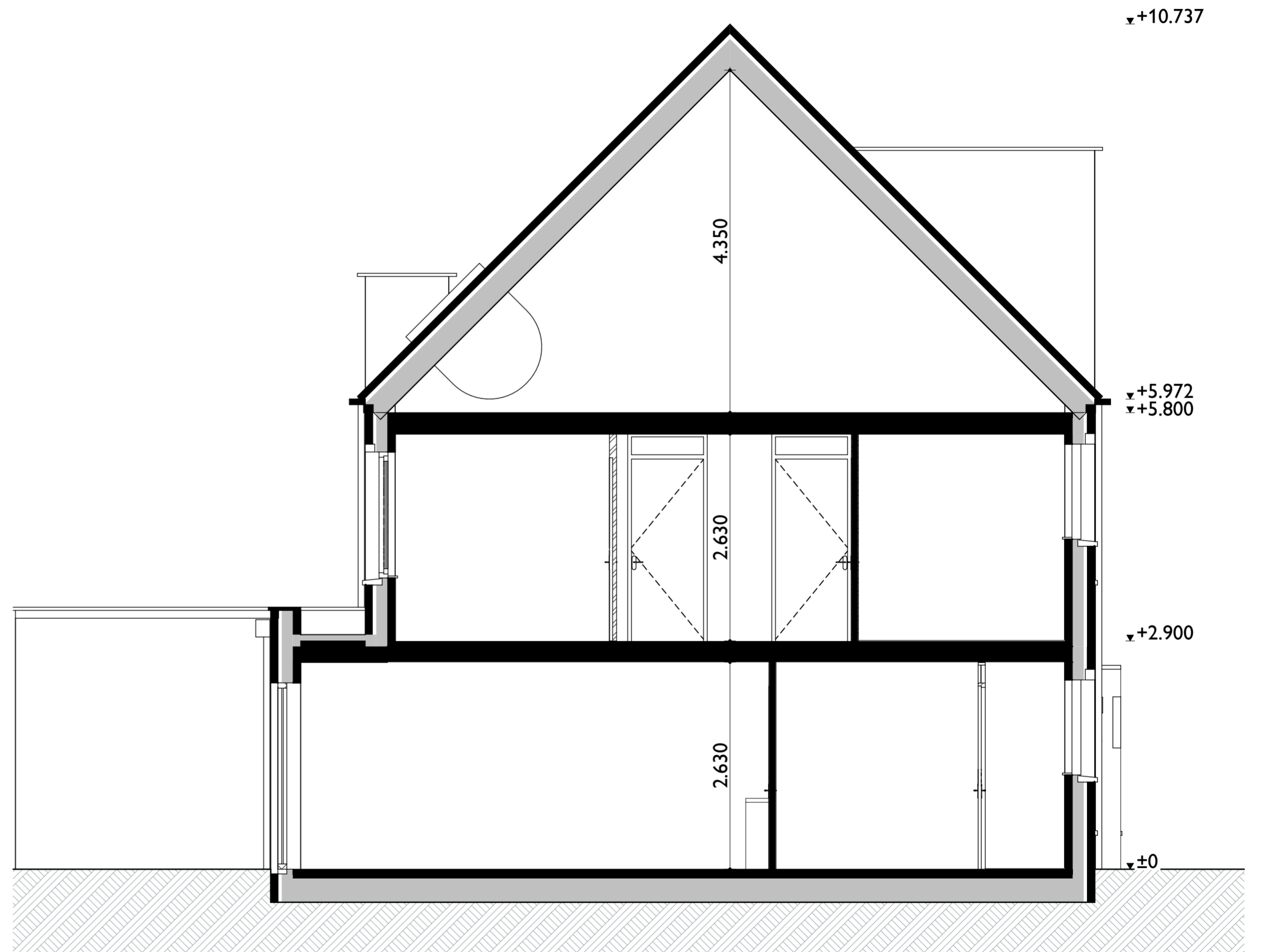
Doorsnede
