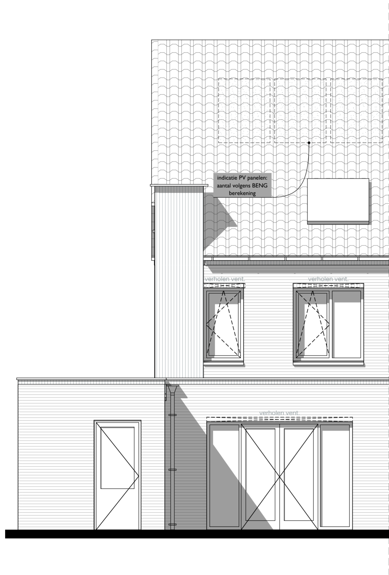
Achtergevel
