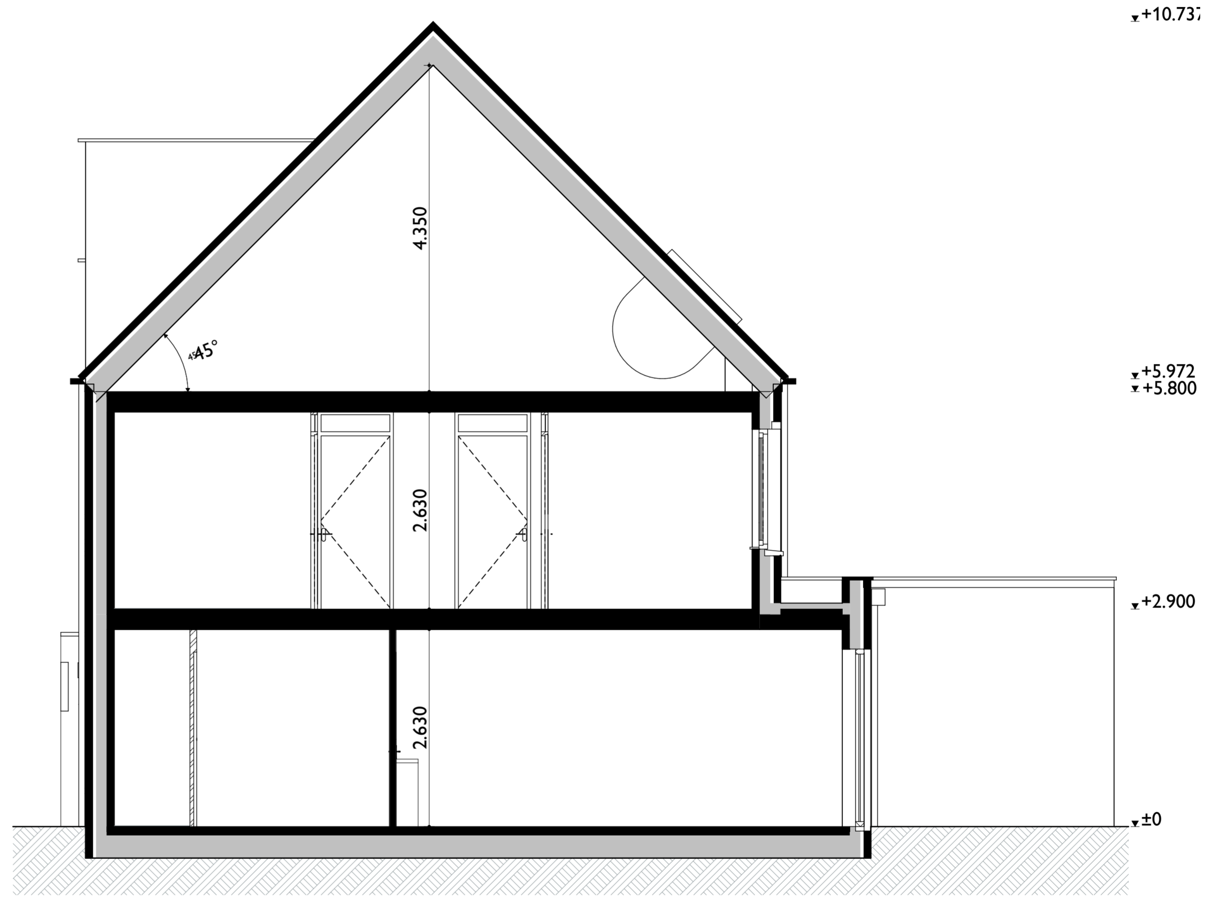
Doorsnede
