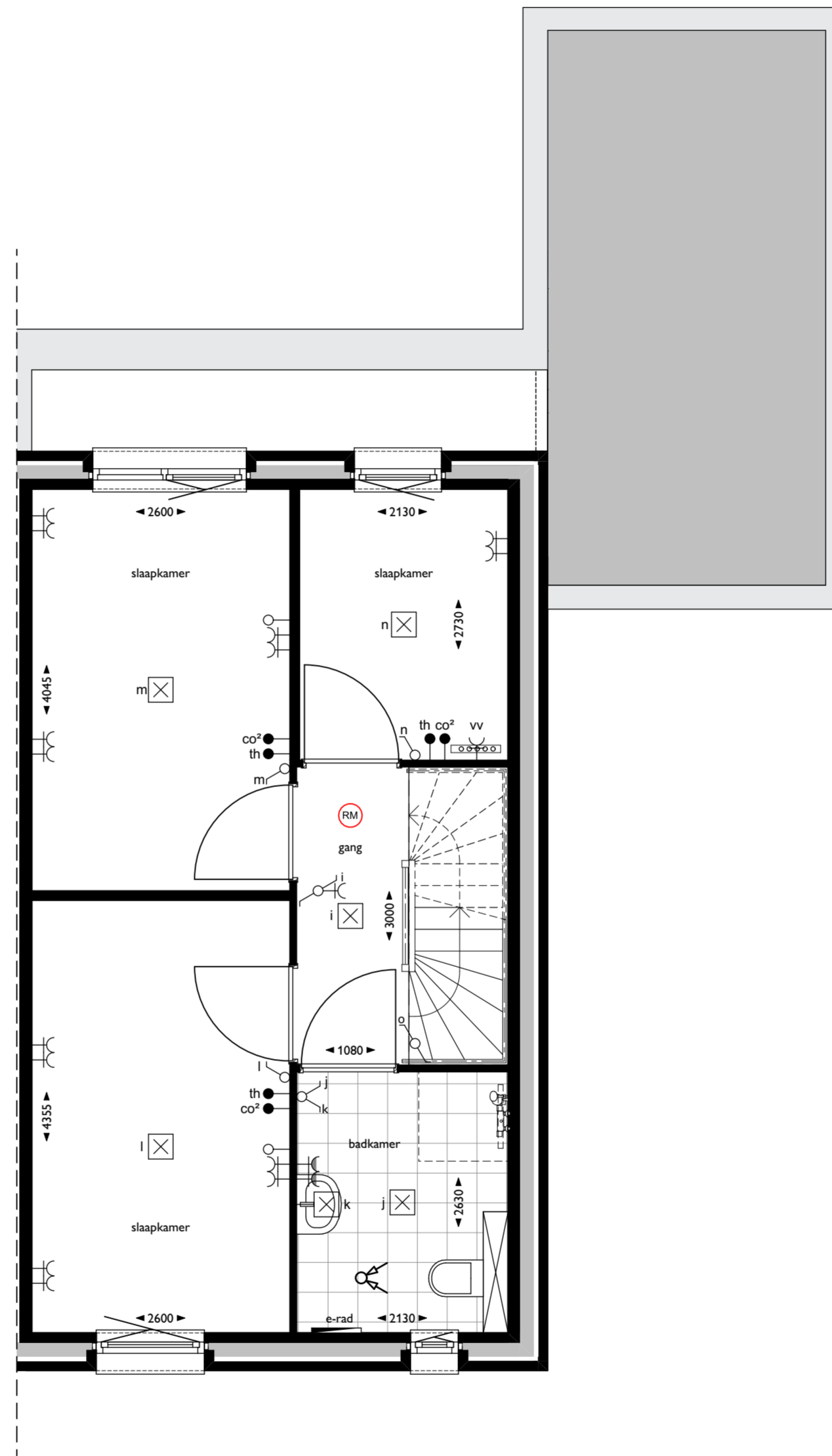
01 eerste verdieping
