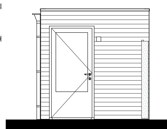
rechter gevel - Berging dubbel hoek
