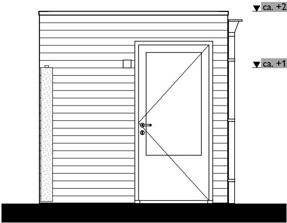
linker gevel - Berging dubbel tussen
