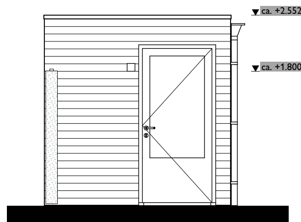
linker gevel - Berging dubbel hoek
