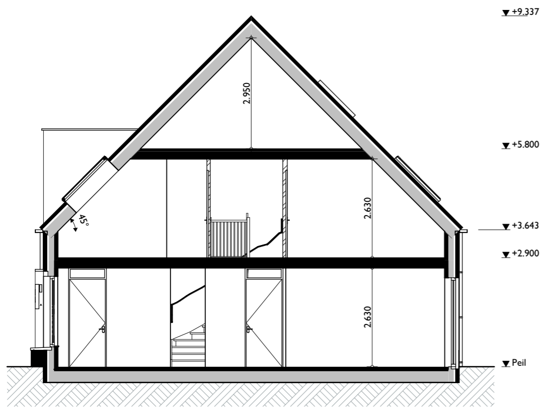
Doorsnede tussenwoning
