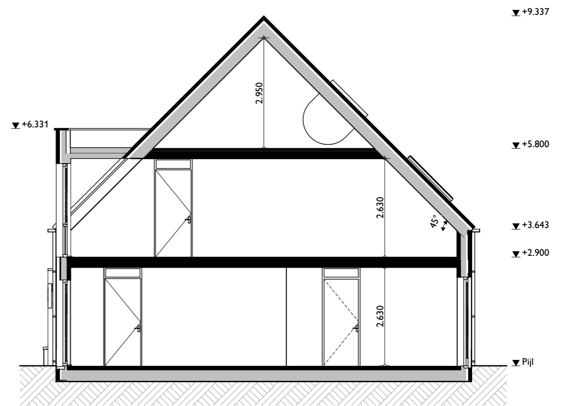
Doorsnede kopwoning
