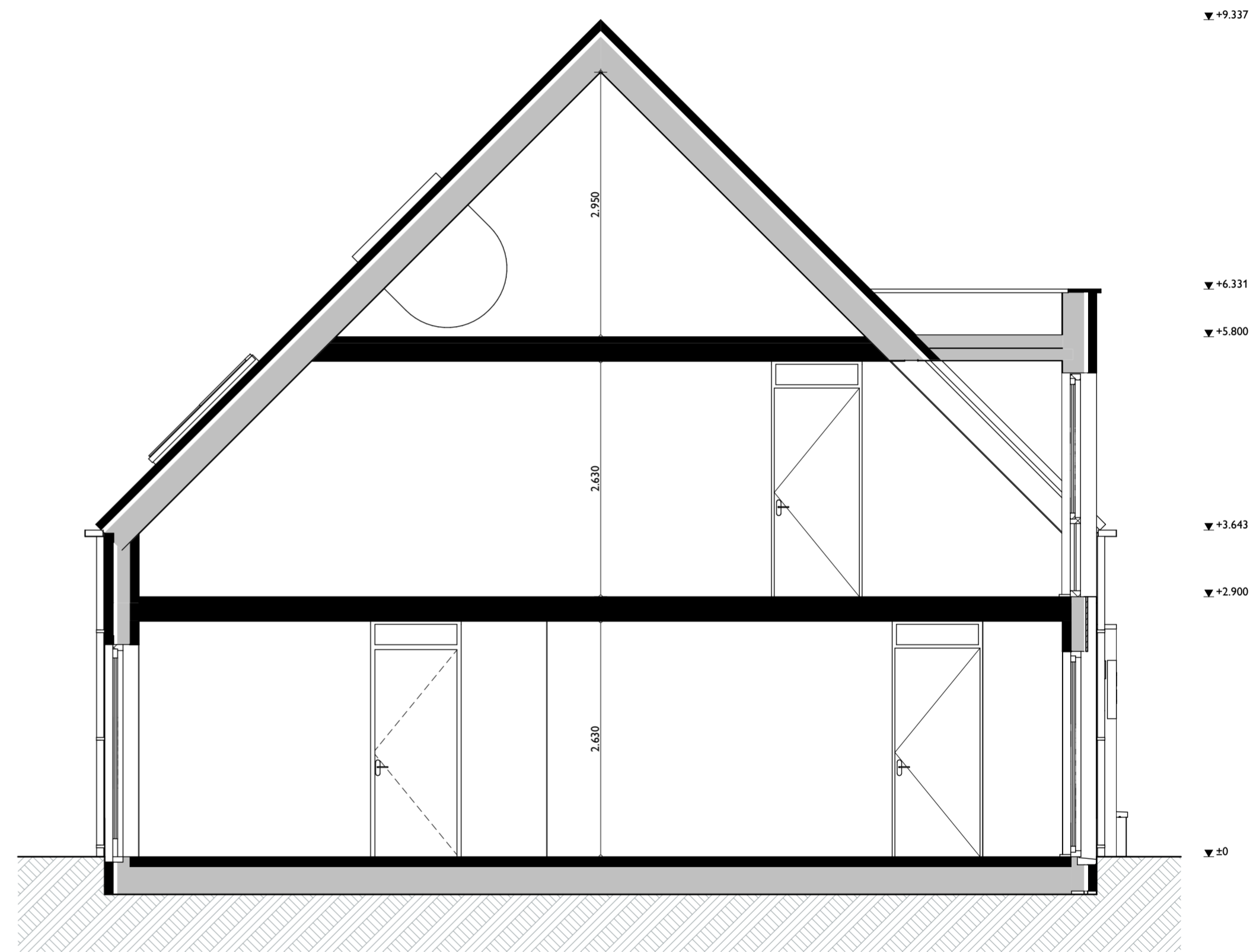
Doorsnede
