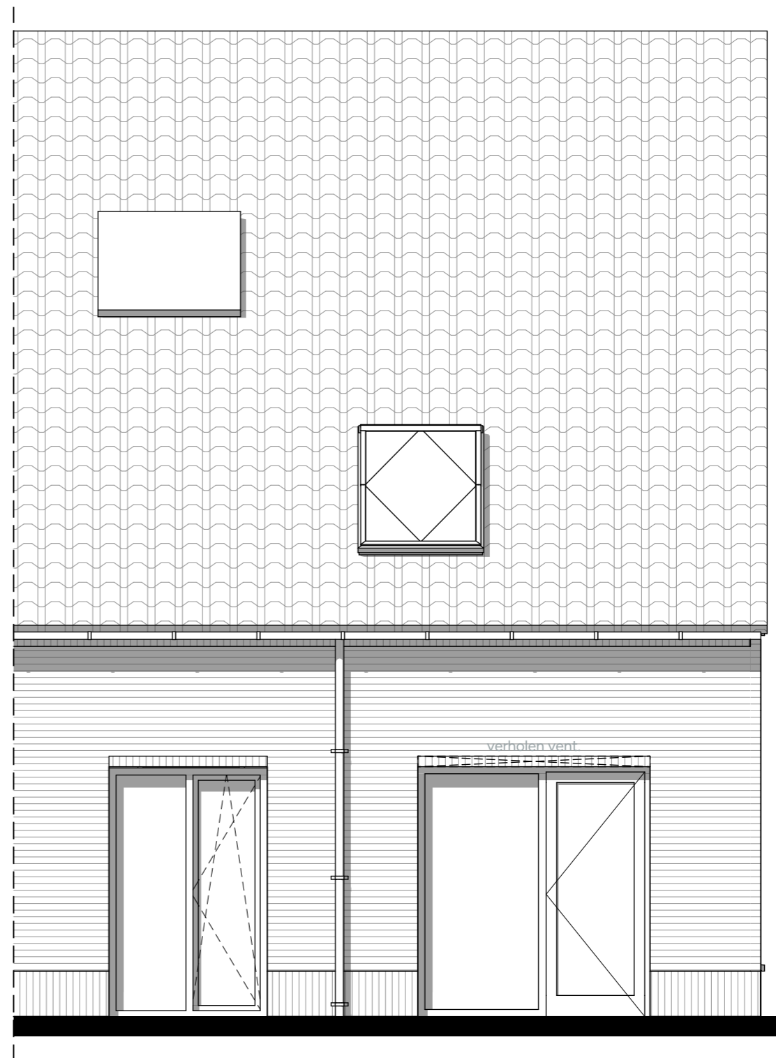
Achtergevel
